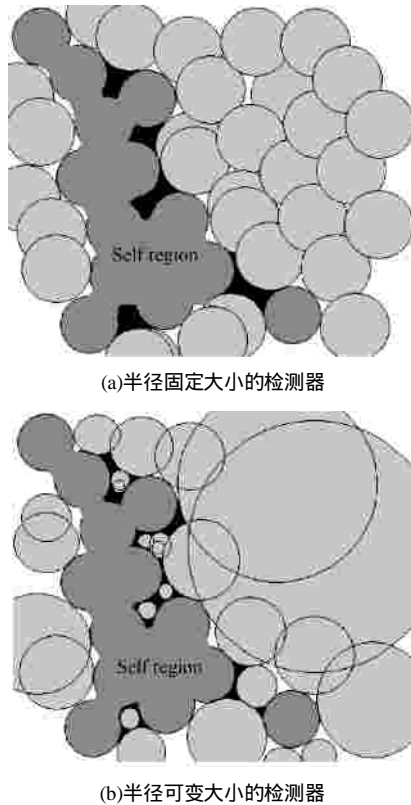
图 6 检测器对比
